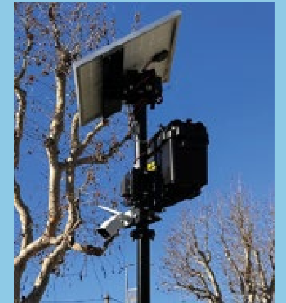
Vidéosurveillance
